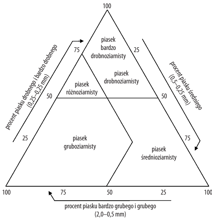
Diagramm kategorien ziarnistości piasków i glin piaszczystych
